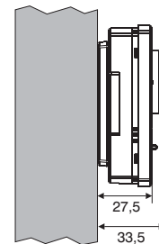
Fernsonde
