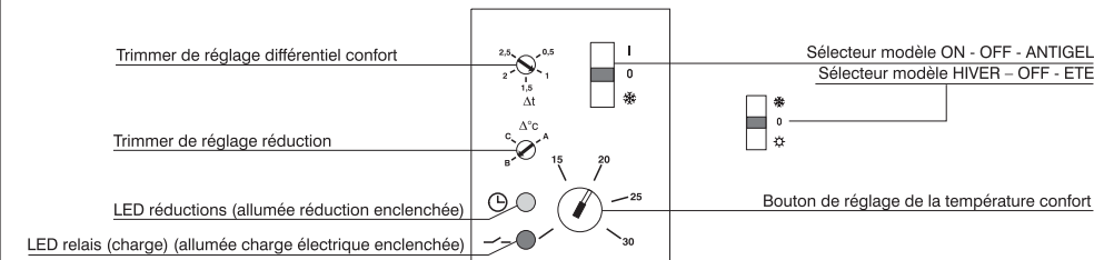
fig. 5 NOTE: Δt = différentiel de température - Δ°C = réduction de la température durant les périodes OFF programmées par l'intermédiaire de l'horloge.
