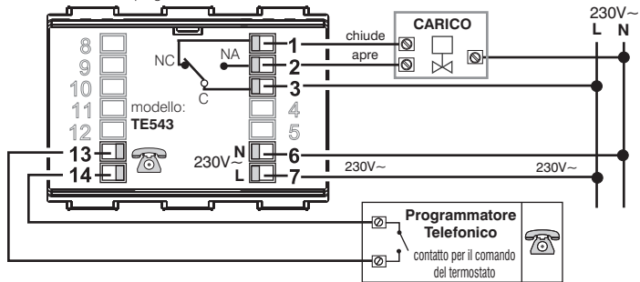
Collegamento ad una valvola motorizzata e ad un programmatore telefonico
